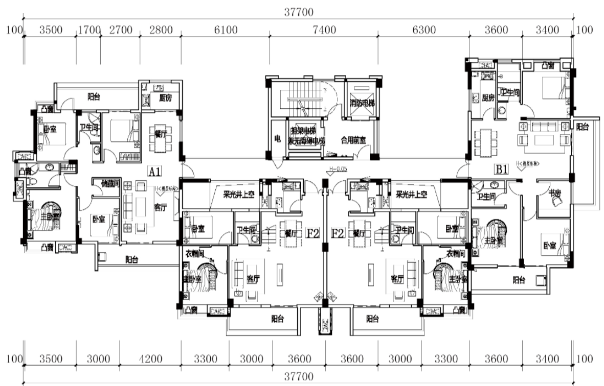
3、1#15 层、2#18 层、3#18 层原户型图
